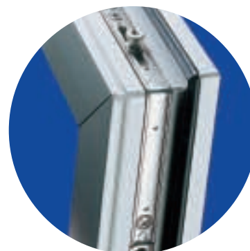
Sicherheitseckumlenkung – serienmäßig beim Standardbeschlag.
